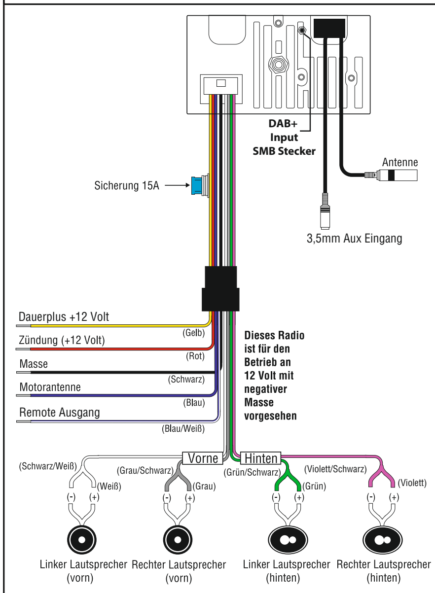
Abbildung 7 - Kabelplan
