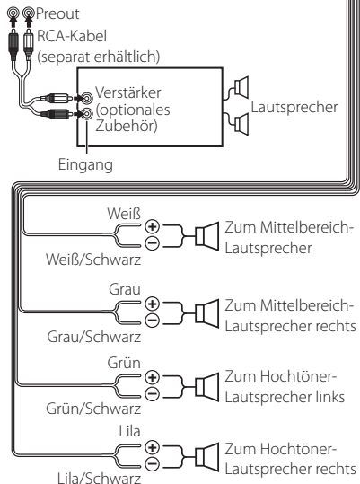
Lautsprecherimpedanz: 4-8 Ω
