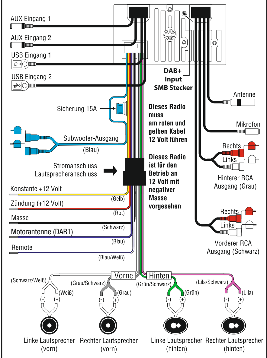
Abbildung 7 - Kabelplan
